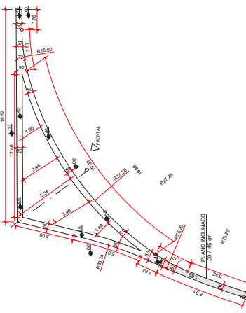
BANCO / JARDINEIRA 1 PLANTA esc. - 1:125
