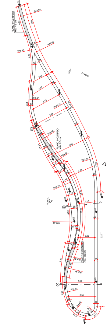
BANCO / JARDINEIRA 2 PLANTA esc. - 1:125
