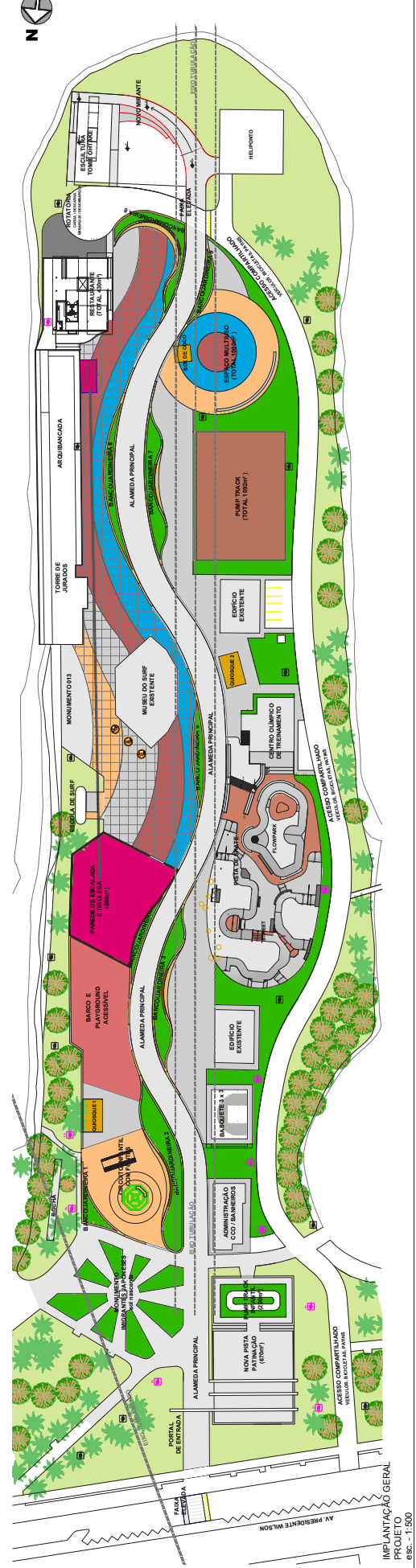
IMPLANTAÇÃO GERAL DIVISÃO DOS MUNDOS - KIDS, RADICAL E 013 esc. - 1:500
