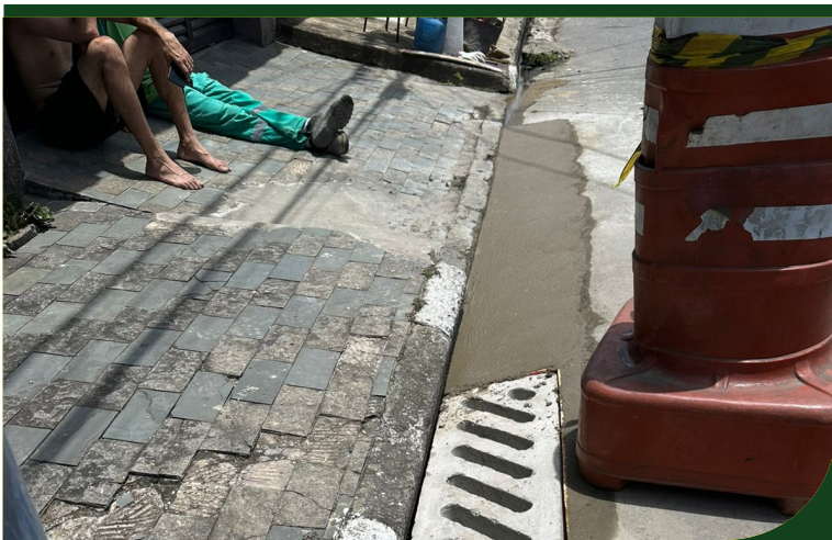
Renivelamento de quatro metros de sarjeta e substituição de boca de lobo
