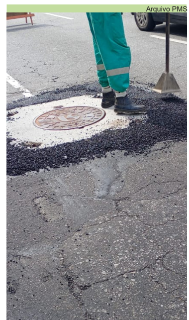
Reparo com massa fria em torno da laje com poço de visita, na Av. Pres. Wilson, sentido Ponta da Praia
