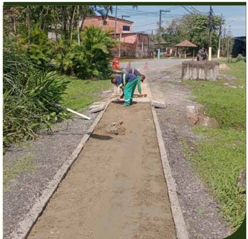
Instalação de placas drenantes no caminho, ao lado da ponte no Monte Cabrão
